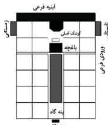
شکل ۴. هندسه باغ ایرانی (مأخذ: پیرنیا، ۱۳۷۳)
